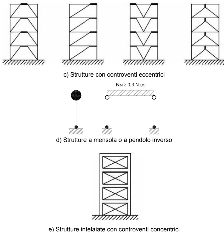
Fig. 7.5.1. - Tipologie strutturali
